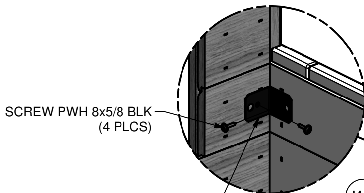
90° L-BRACKET - BLK (2 PLCS)
