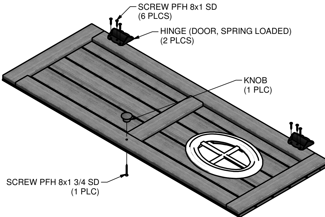
RIGHT SIDE DOOR ASSEMBLY
