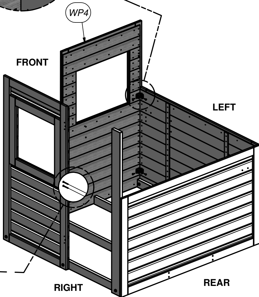
90° L-BRACKET - BLK (2 PLCS)
